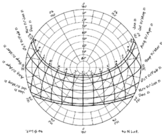
Sun Path Diagram, 36° Latitude
