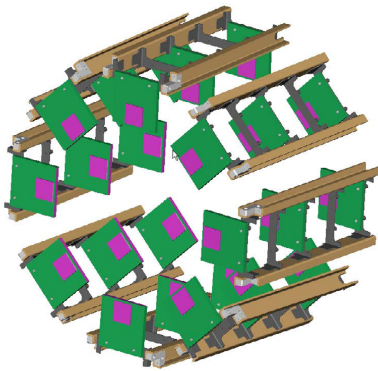
PLT Telescope Array
