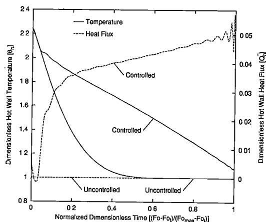
(d) \theta_i = 2.391 , Fo_l = 0.247 , G_{ld}^L = 1.247 .
