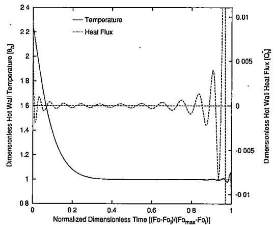
(d) \theta_i = 2.391 , Fo_i = 0.247 , G_{L_d}^L = 1.103 .
