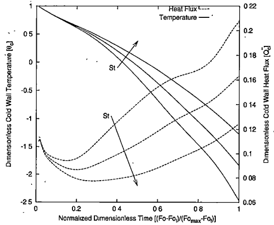
(d) \theta_i = 2.391 , Fo_i = 0.247 , and G_{l_d}^L = 1.558 .
