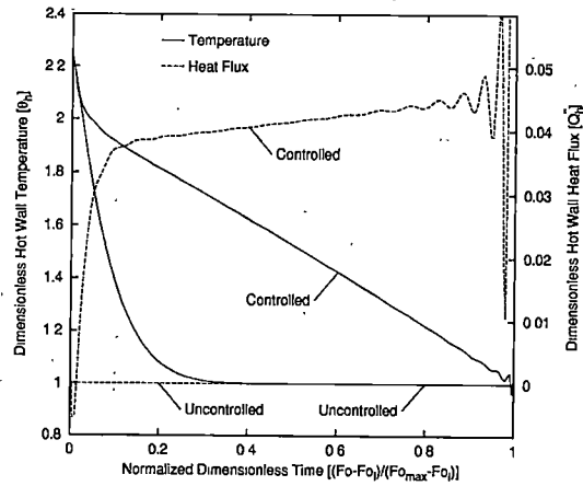
(d) \theta_i = 2.391 , Fo_l = 0.247 , and G_{ld}^L = 1.103 .
