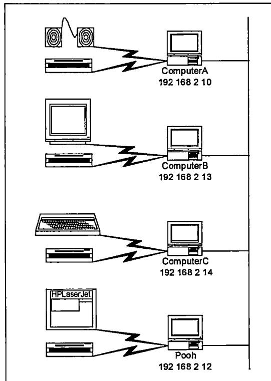
Figure 5 2 Actual system
