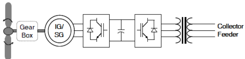
(d) Type 4 WECS
