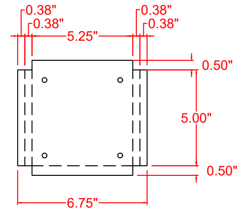
Unbent Piece
