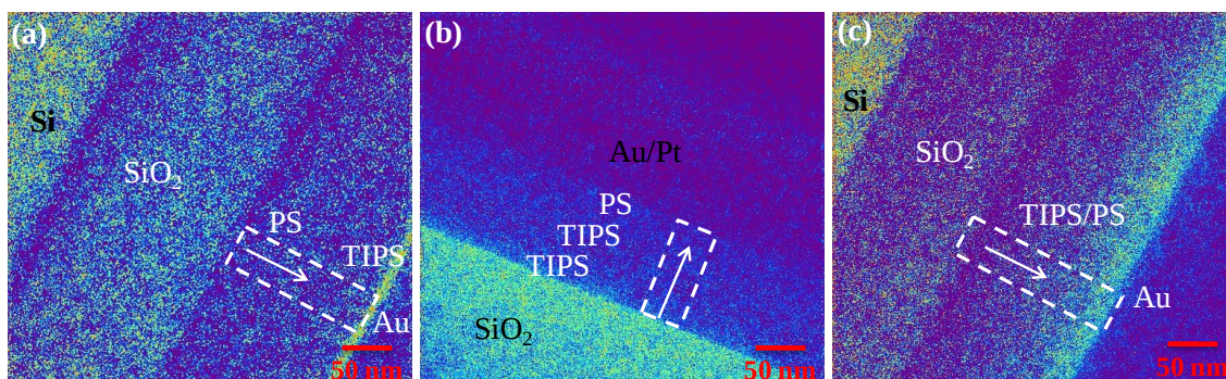
Figure 8.7. Cross-section EFTEM images for a) TIPS-PEN:4-arm star PS, b) TIPS-PEN:linear PS, and c) TIPS-PEN:centipede PS films.
