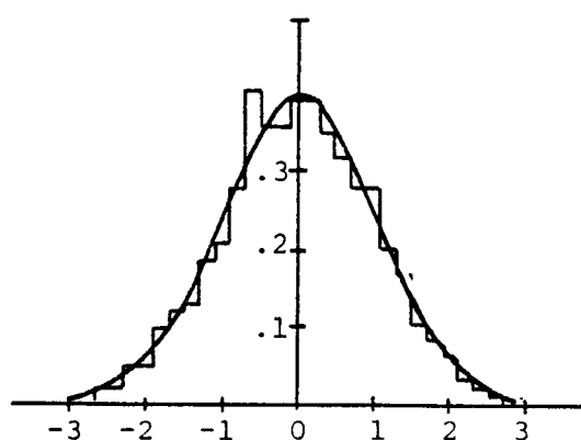
(d) Simulated turbulence of approximate von Karman model
