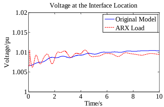
(d) Voltage at the Interface Location
