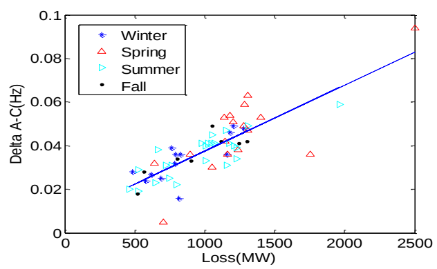
(d) Inertial frequency response vs. MW loss
