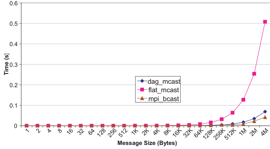
(d) 32 Processes
