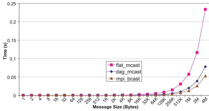
(d) 32 Processes
