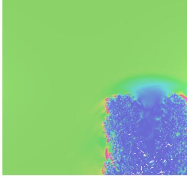
(d) t = 288.0 \mu s , (22.40 MPa), Before Material Failure
