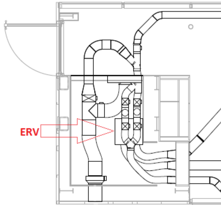
Fig. 4.2. ERV Ductwork
