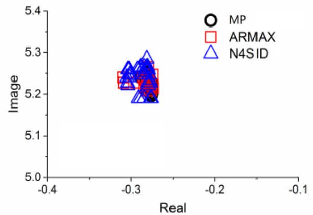
(d) Mode 4(0.83Hz)
