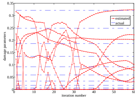
Fig. 3.26-b Estimated shaft damage parameters vs. iteration number; symmetric AMB mass tuning set, AMB location x = 0.375L , \Omega = 900 RPM.
