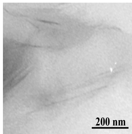
Cloisite 25A
