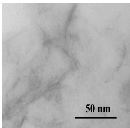
Cloisite Na +
