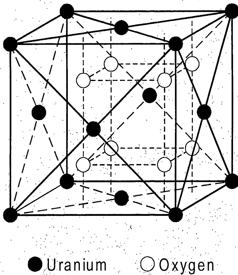
Fig. 2.2. Crystal structure of UO 2 (Katz 1986).
