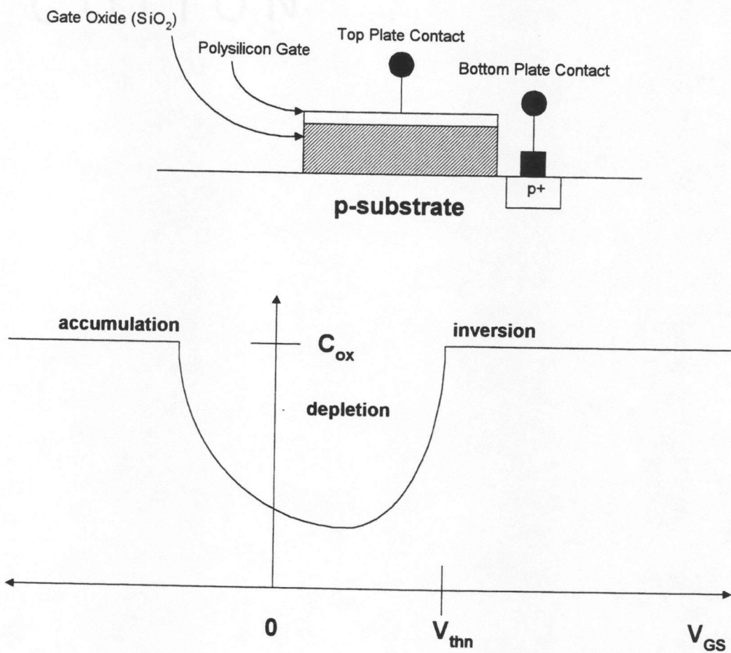
Figure 13 - Simple MOS IC Capacitor
