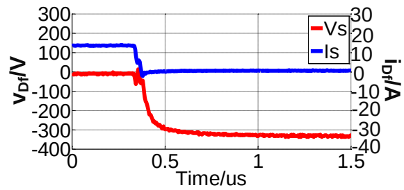
(d) Df turn-off transition
