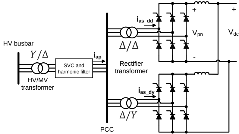
Fig. 1-3. 12-pulse thyristor rectifier.
