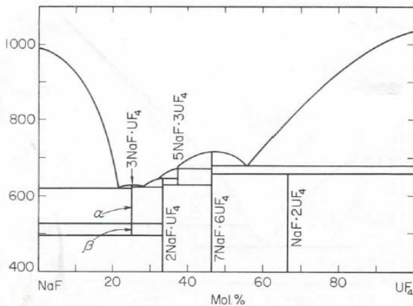
FIG. 1498.—System NaF-UF 4 .
