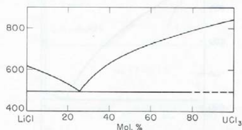
FIG. 1297.—System LiCl-UCl 3 .
