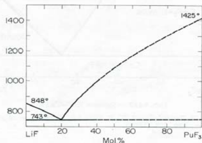
FIG. 1475.—System LiF-PuF 3 .
