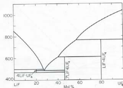
FIG. 1479.—System LiF-UF 4 .
