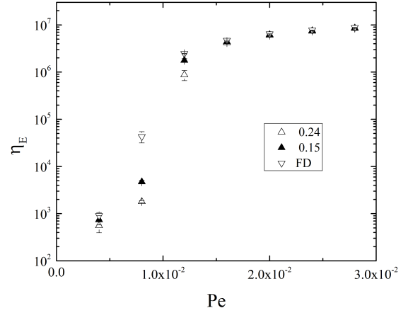
(d) R44, b = 5000
