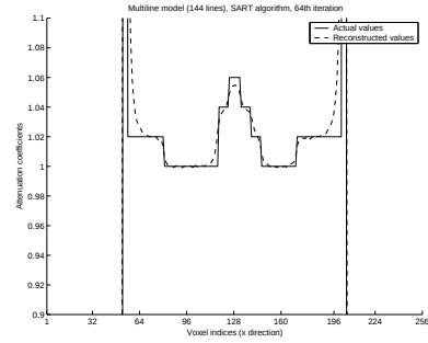
(b) Multiline/SART
