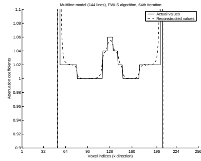
(f) Multiline/FWLS
