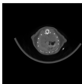
(d) Multiline/EM
