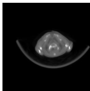
(f) Multiline/FWLS
