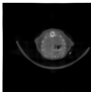
(b) Multiline/SART
