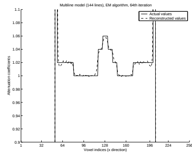
(d) Multiline/EM
